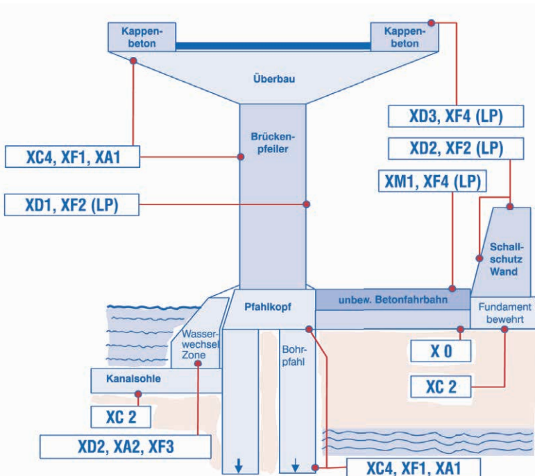
Beispiele für Beton im Industriebau. Für die richtige Auswahl der Betonsorte, ist allein der Abnehmer verantwortlich.
