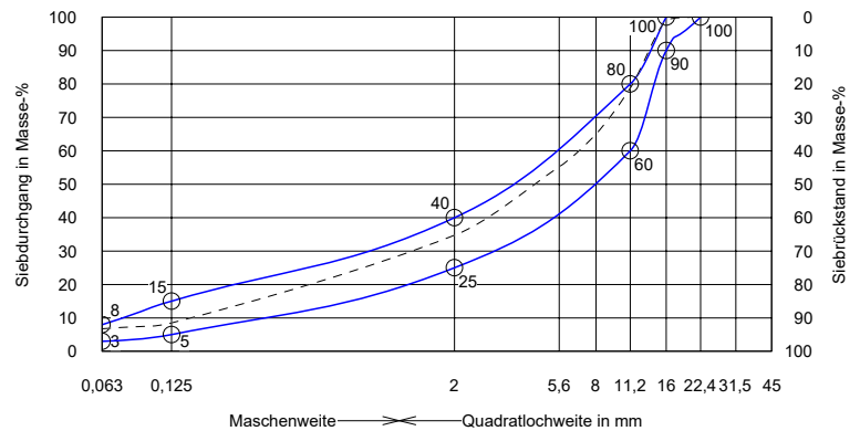
Sieblinienbereich für AC 16 B N
